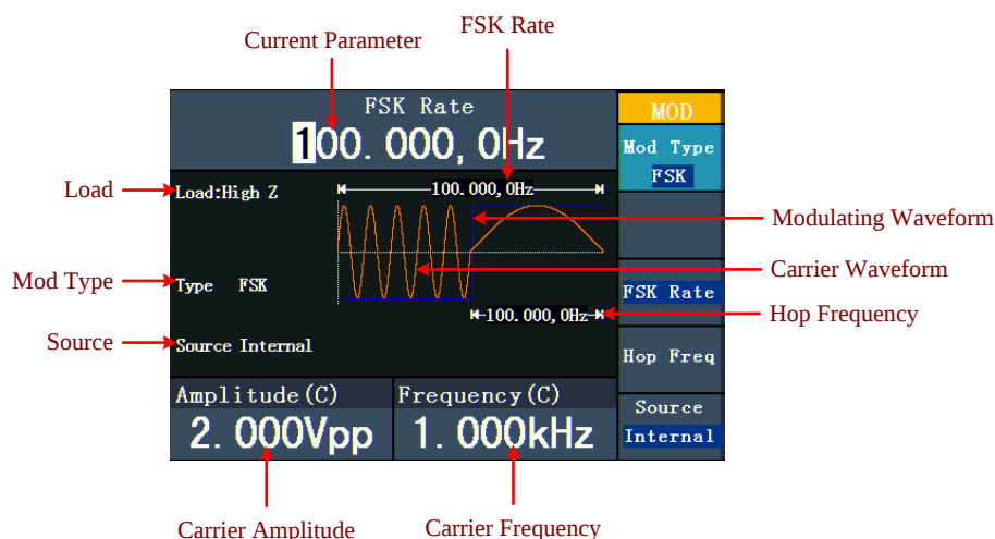
Rys. 0-19: Interfejs użytkownika FSC
