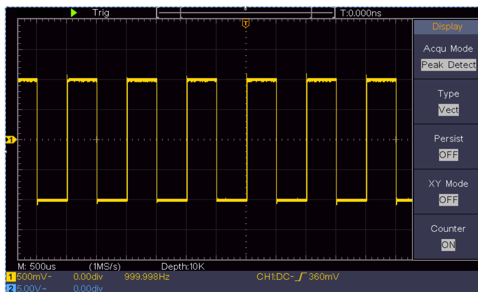
Figura 0-4 Segnale con rumori
