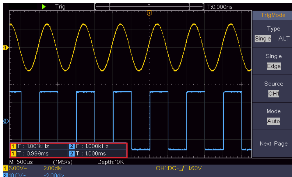
Figura 0-1 Misurare il periodo e il valore della frequenza per un dato segnale
