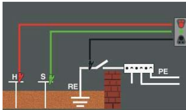
Esquema de configuración para la medición de resistencia de tierra (RE)
