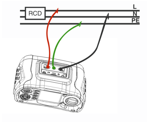
Anschluss bei der FI-Messung
