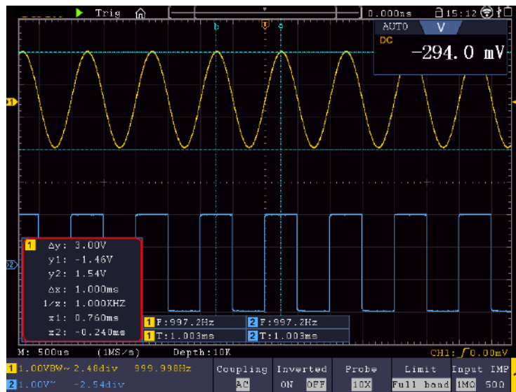
Figure 4.14 Mesure du curseur de temps et de tension
