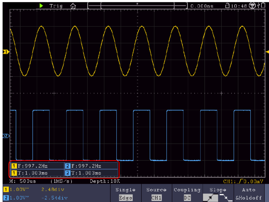
Figure 4.11 Mesure automatique
