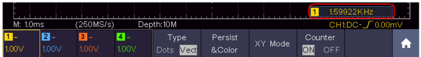
Figure 4.5 Affichage du compteur de fréquence 4CH
