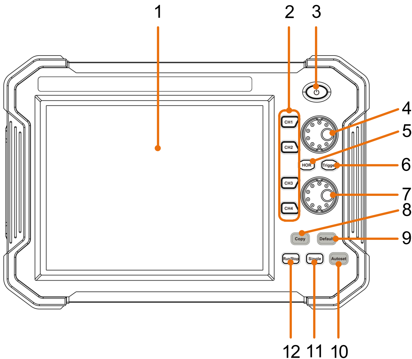
Figure 1.0 Vue avant (Oscilloscope 4 voies)
