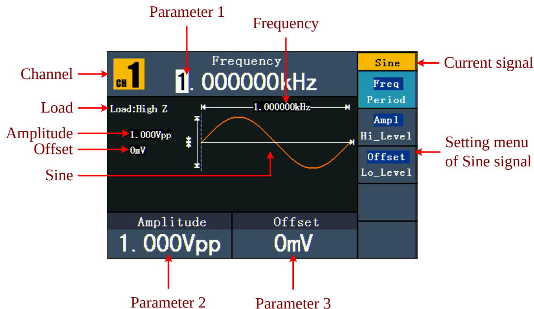
Fig. 0-5 : L'interface utilisateur du signal sinusoïdal
