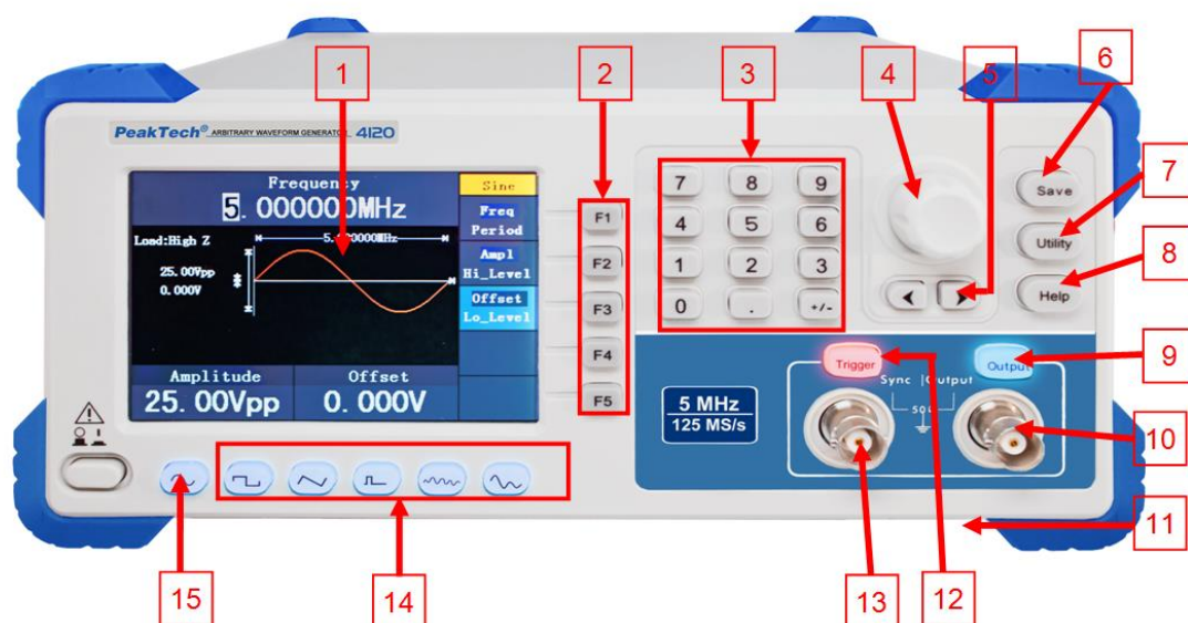
Fig. 0-1 Vue d'ensemble du panneau de commande
