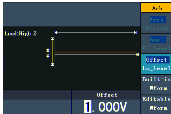
Fig. 0-15 : L'interface de réglage du CC
