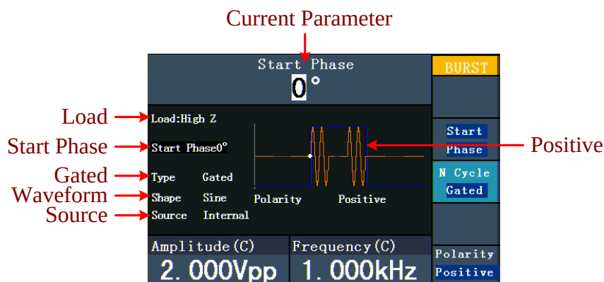
Fig. 0-22 : L'interface utilisateur de Gated Burst
