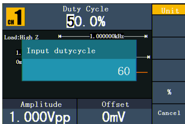
Fig. 0-8 : Réglage du rapport cyclique d'un signal rectangulaire
