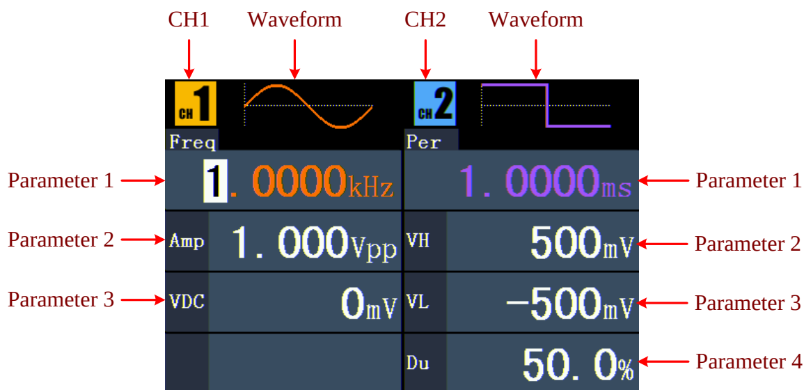
Fig. 0-4 : L'interface utilisateur du bouton "Les deux".
