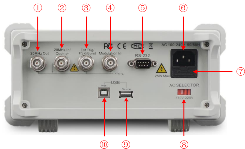
Fig. 0-2 Vue d'ensemble du dos
