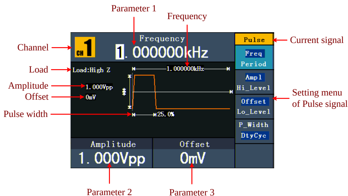
Fig. 0-11 : L'interface utilisateur du signal d'impulsion
