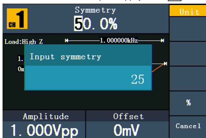
Fig. 0-10 : Réglage de la symétrie du signal de rampe
