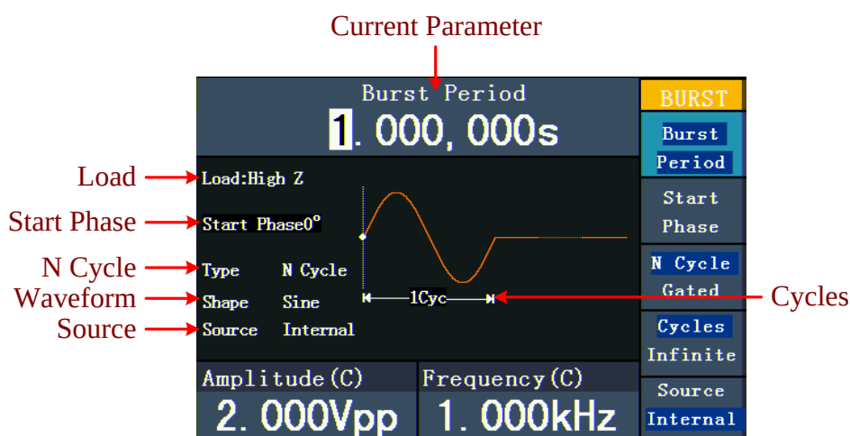
Fig. 0-21 : L'interface utilisateur de N-Cycle-Burst
