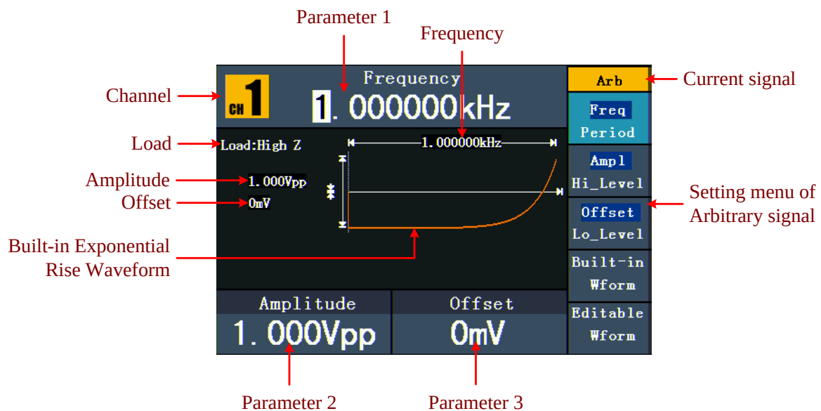
Fig. 0-14 : L'interface utilisateur du signal arbitraire
