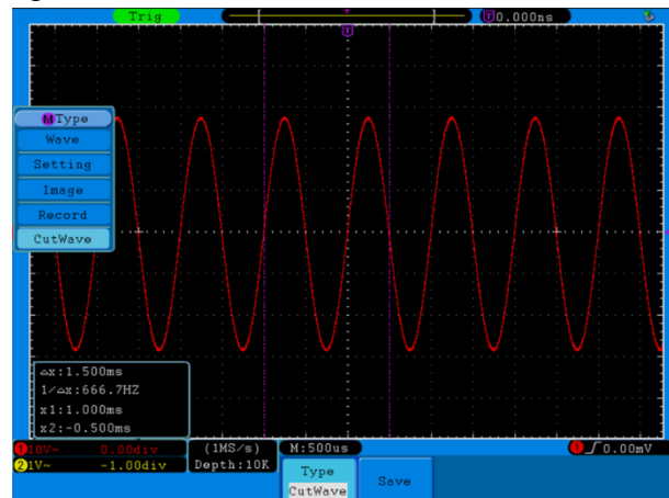
Fig. 0-24 : Onde de coupe (coupe de la forme d'onde)
