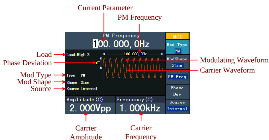
Fig. 0-18 : L'interface utilisateur du PM
