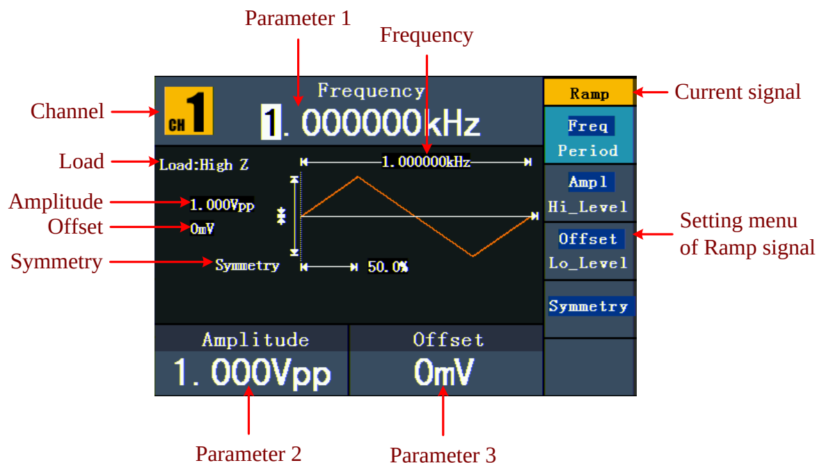
Fig. 0-9 : L'interface utilisateur du signal de rampe
