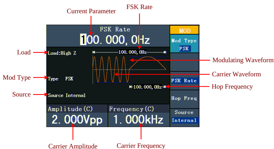
Fig. 0-19 : L'interface utilisateur du FSC
