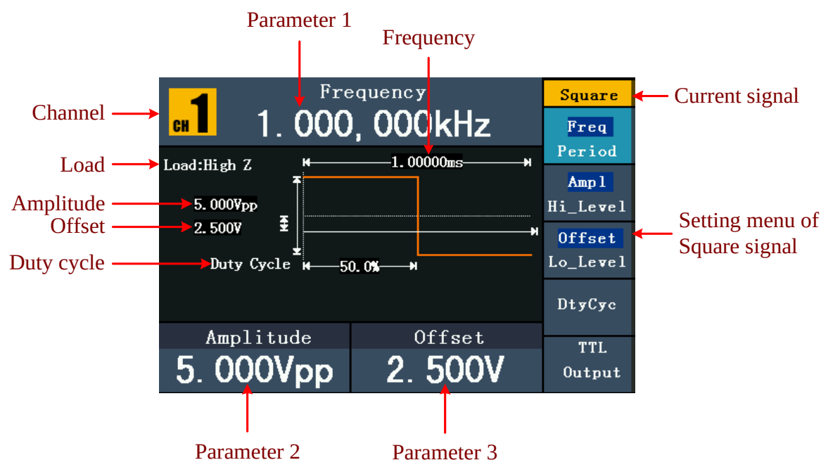
Fig. 0-7 : L'interface utilisateur du signal d'onde carrée
