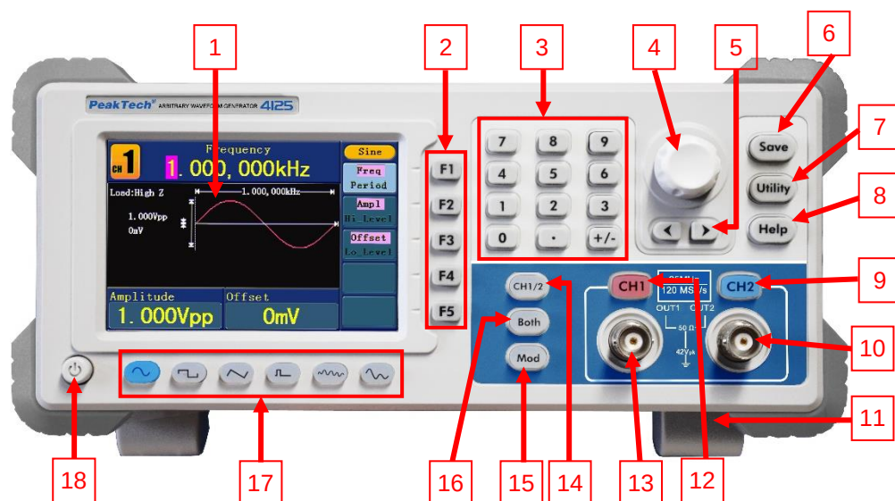
Fig. 0-1 Vue d'ensemble du panneau de commande
