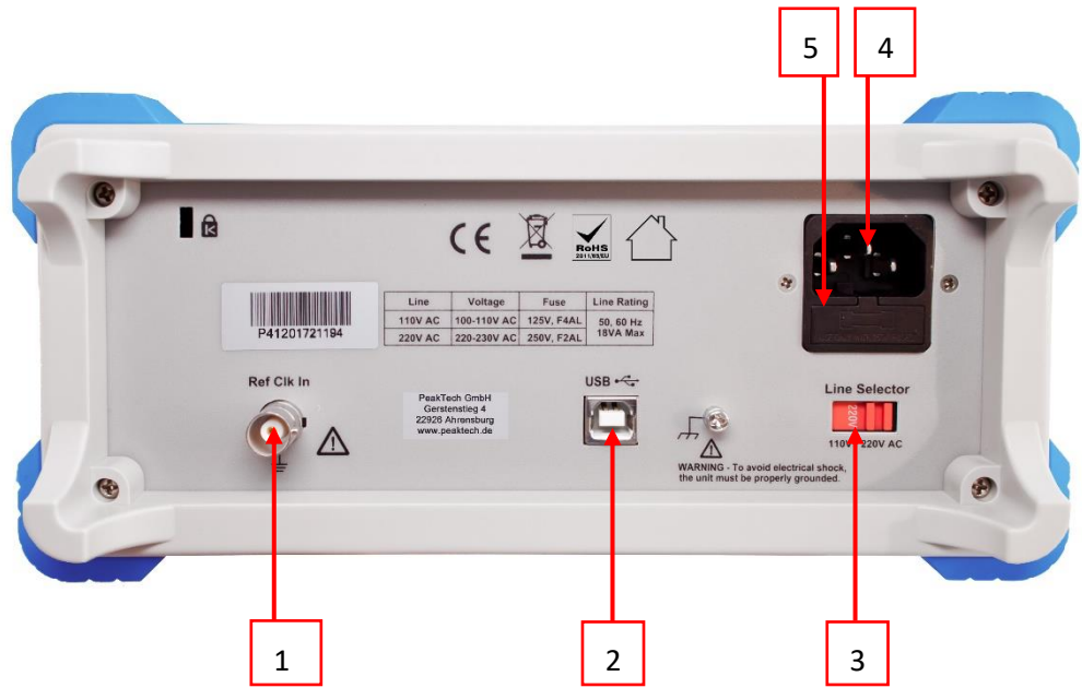
Fig. 0-2 Vue d'ensemble du dos
