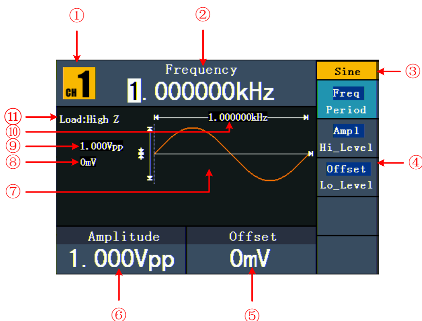
Fig. 0-3 Interface utilisateur (par exemple, sinus)
