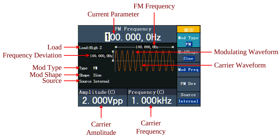
Fig. 0-17 : L'interface utilisateur du FM
