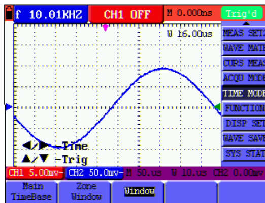
Abbildungen 62: Fenstervergrößerung
