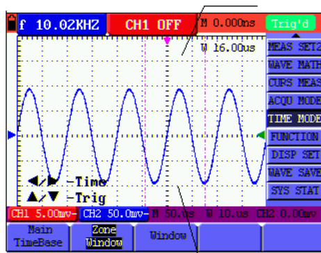
Abbildung 61: Fenstereinstellungen
