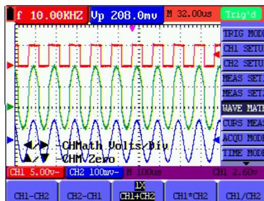
Abbildung 18: Kurven-Rechenfunktion
