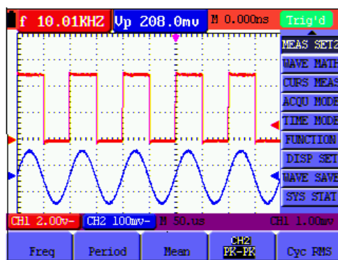
Abbildung 49: Automatische Messungen
