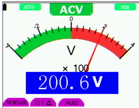
Abbildung 26: Wechselspannungsmessung (ACY)
