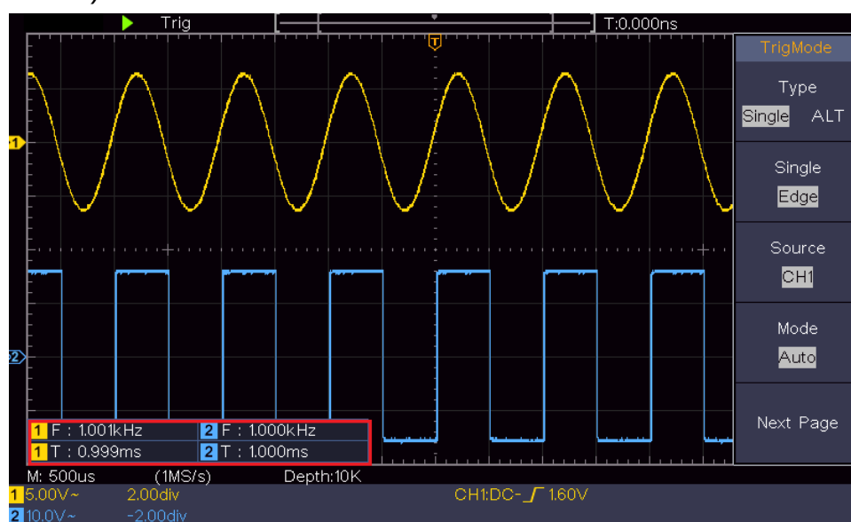
Figure 3-13 Mesure automatique
